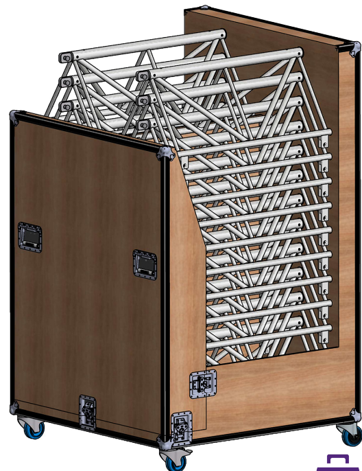
Abmessungen: 119x119x196 cm (LxBxH)
