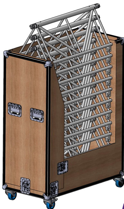
Abmessungen: 119x59x190 cm (LxBxH)
